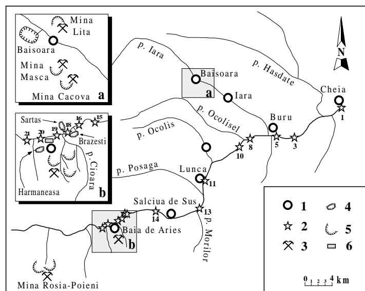
Fig. 1. Principalele zone miniere din perimetrul studiat, care contribuie la poluarea râului Arieș. 1 – localități; 2 – puncte de probare; 3 – mine; 4 – iazuri de decantare; 5 – halde de steril; 6 – uzină de preparare a minereului.
