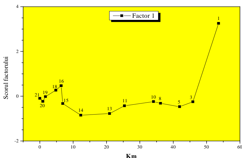
Fig. 3. Variația scorului factorului 1 între localitățile Muncel și Cheia. Numerele reprezintă punctele de prelevare a probelor.
